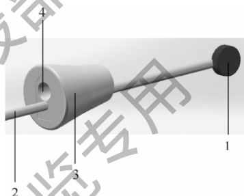
图 B.1.1 传感器示意
