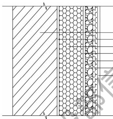
图 6.6.1 现场喷涂硬泡聚氨酯外保温系统
